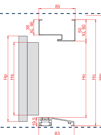
DUOTHERM 75
