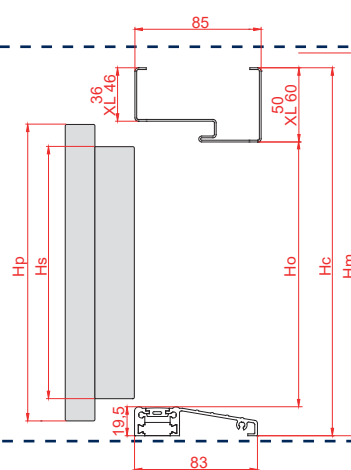
DUOTHERM 60
