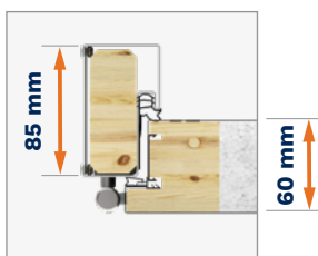
Ościeżnica DUOTHERM 60
